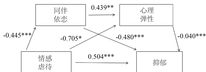
Figure 1. The mediating role of peer attachment and resilience 图 1. 同伴依恋和心理弹性的中介作用示意图
