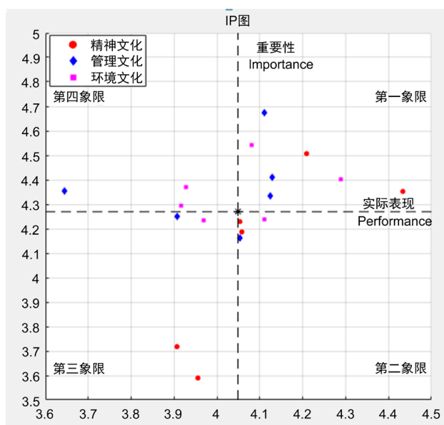
Figure 2. Shows the position of the vertical intersection of the I value and the P value of each indicator variable in the IP map 图 2. 各指标变量的 I 值与 P 值垂直交点在 IP 图中的位置显示
