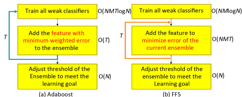
Figure 4. The comparison of Adaboost and FFS 图 4. Adaboost 和 FFS 比较
