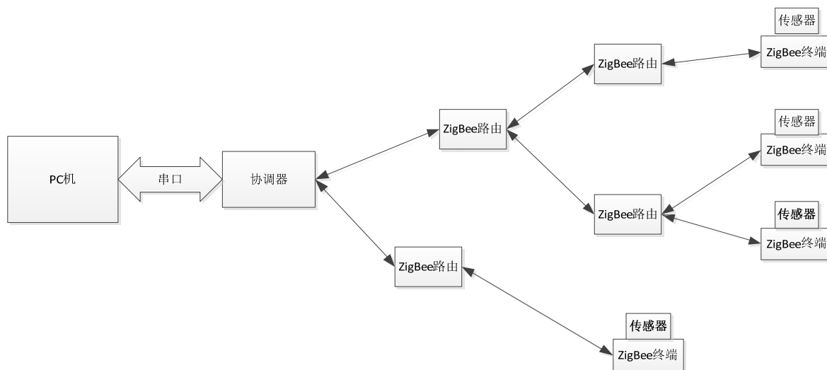
Figure 1. System Structure 图 1. 系统结构框图
