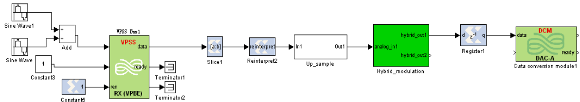
Figure 10. System transmitter block diagram in Simulink 图 10. Simulink 中发射系统结构图
