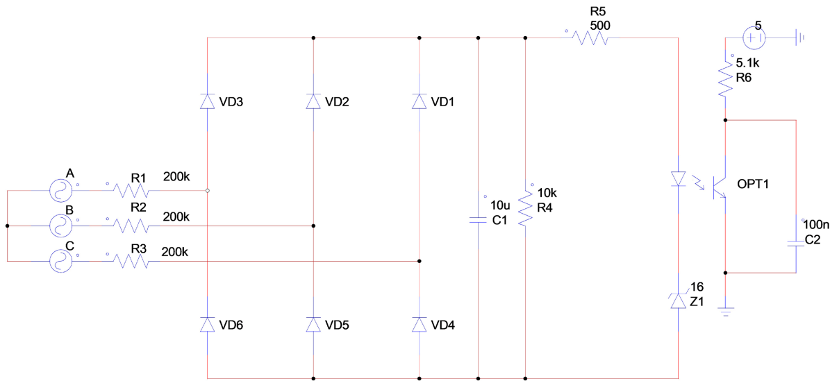
Figure 11. Simulation schematic 图 11. 仿真原理图
