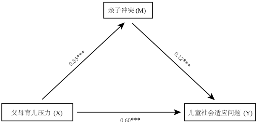
Figure 1. Correlation diagram of dimensions 图 1. 各维度相关性图
