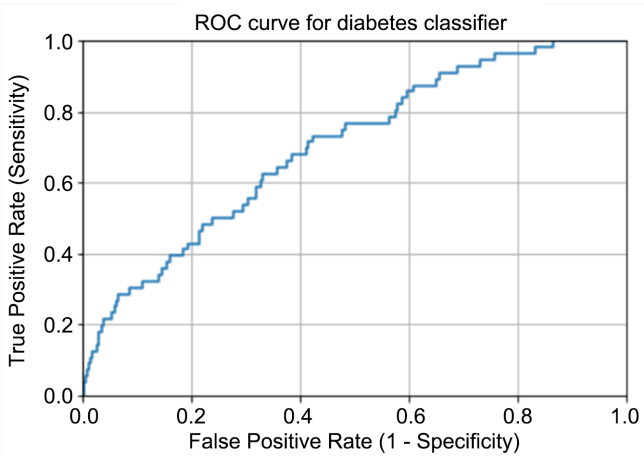
Figure 3. ROC curve 图 3. ROC 曲线图
