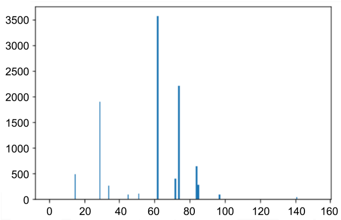
Figure 7. CATBoost indicator importance histogram 图 7. CATBoost 指标重要性柱状图
