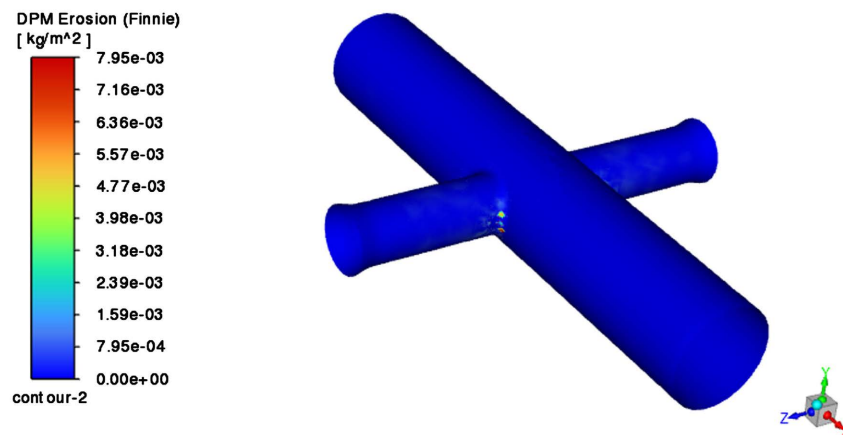
Figure 5. Cloud map of pipe wall erosion 图 5. 管壁冲蚀云图
