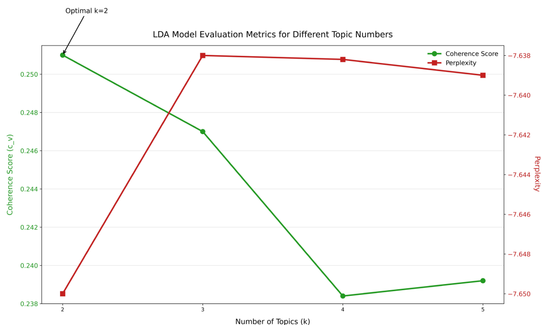
Figure 2. LDA model evaluation metrics 图 2. LDA 模型评估指标变化
